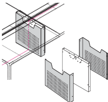
Pannello carter per gamba intermedia.
