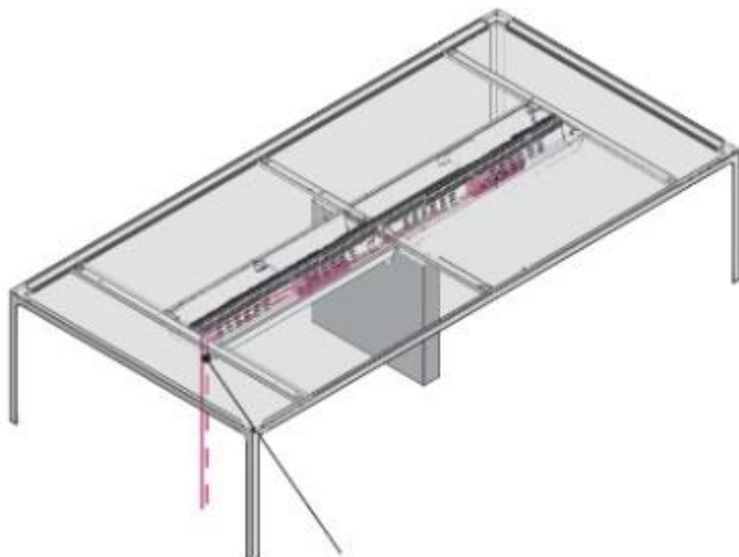
Salita cavi con calza su colonna senza carter.
