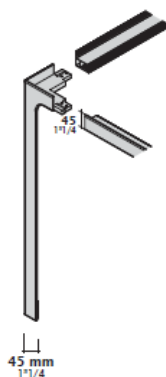
Dettaglio: attacco gamba - profili piano.
